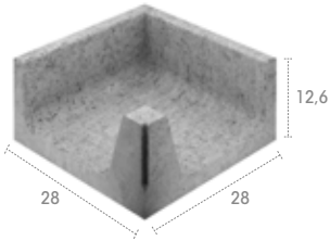
RS 943 Esquina interior Inside corner Angle intérieur
