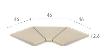
SI3 Anti-Slip 46 x 46 x 2,6
