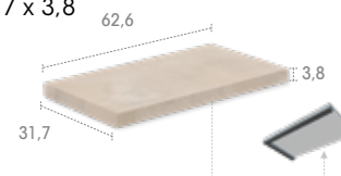
EI6 Anti-Slip 62,6 x 31,7 x 3,8
