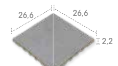
245 EF Anti-Slip 26,6 x 26,6 x 2,2
