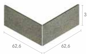
EJ6 Anti-Slip 62,6 x 62,6 x 31
