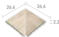
245 EF Anti-Slip 26,6 x 26,6 x 2,2
