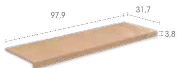
L98 Anti-Slip 97,9 x 31,7 x 3,8
