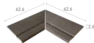
664 Anti-Slip 62,6 x 62,6 x 2,6
